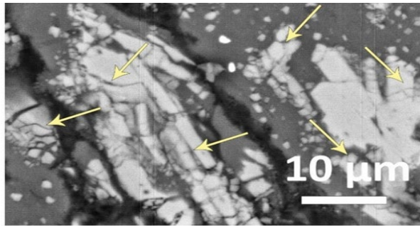
Рис. 5. Крихке руйнування інтерметалідів під час пресування
