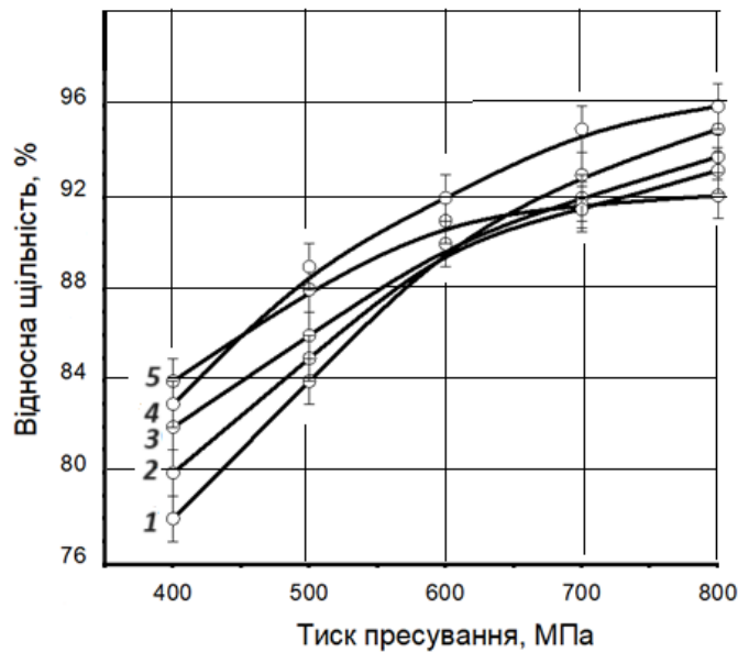
Рис. 3. Залежність відносної щільності зразків Al-15Fe різного фракційного складу від тиску пресування: 1 – 100 мкм ; 2 – 200 мкм; 3 – 282 мкм; 4 – суміш; 5 – 357 мкм
