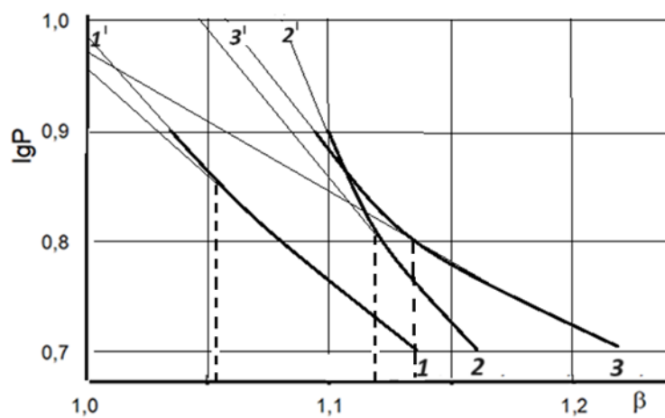
Рис. 4. Залежності LgP - \beta для порошків з різним середнім розміром частинок: 1 – суміш; 2 – 282 мкм; 3 – 100 мкм
